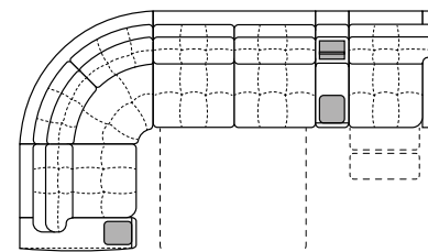
432 см x 255 см Спальное место: 160 см x 200 см Модуль «реклайнер» в положении «релакс»: 80 см x 177 см
