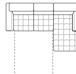
297 см x 195 см Спальное место: 160 см x 197 см
