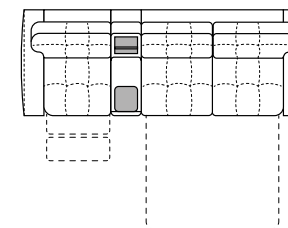
319 см x 120 см Спальное место: 160 см x 200 см Модуль «реклайнер» в положении «релакс»: 80 см x 177 см
